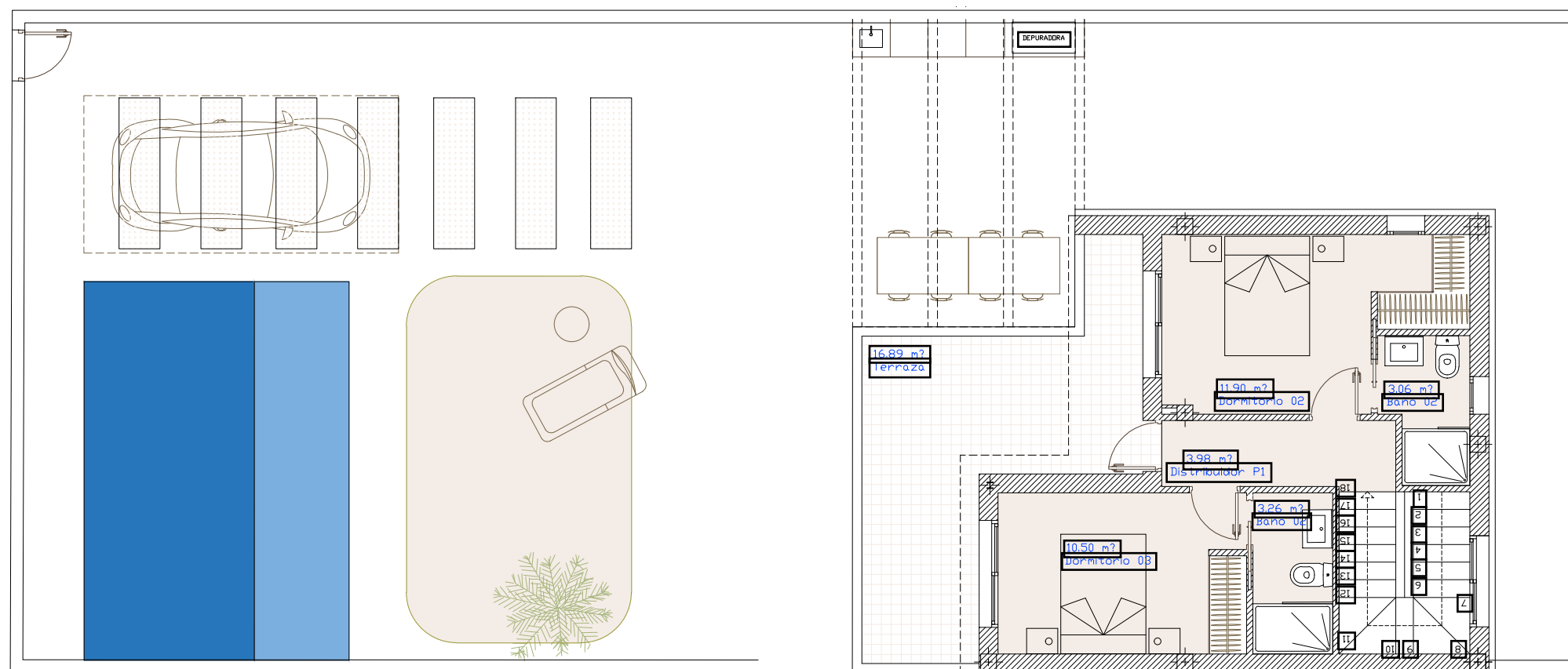
PLANTA PRIMERA
